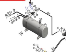
TANQUE HIDRÁULICO SC 190 LITROS ALUMI
