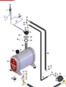
KIT HIDRÁULICO MINERAÇÃO SPEEDY
