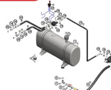
TANQUE HIDRÁULICO SC 190 LITROS SEM OVAL
